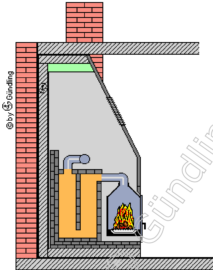
Seitenansicht
